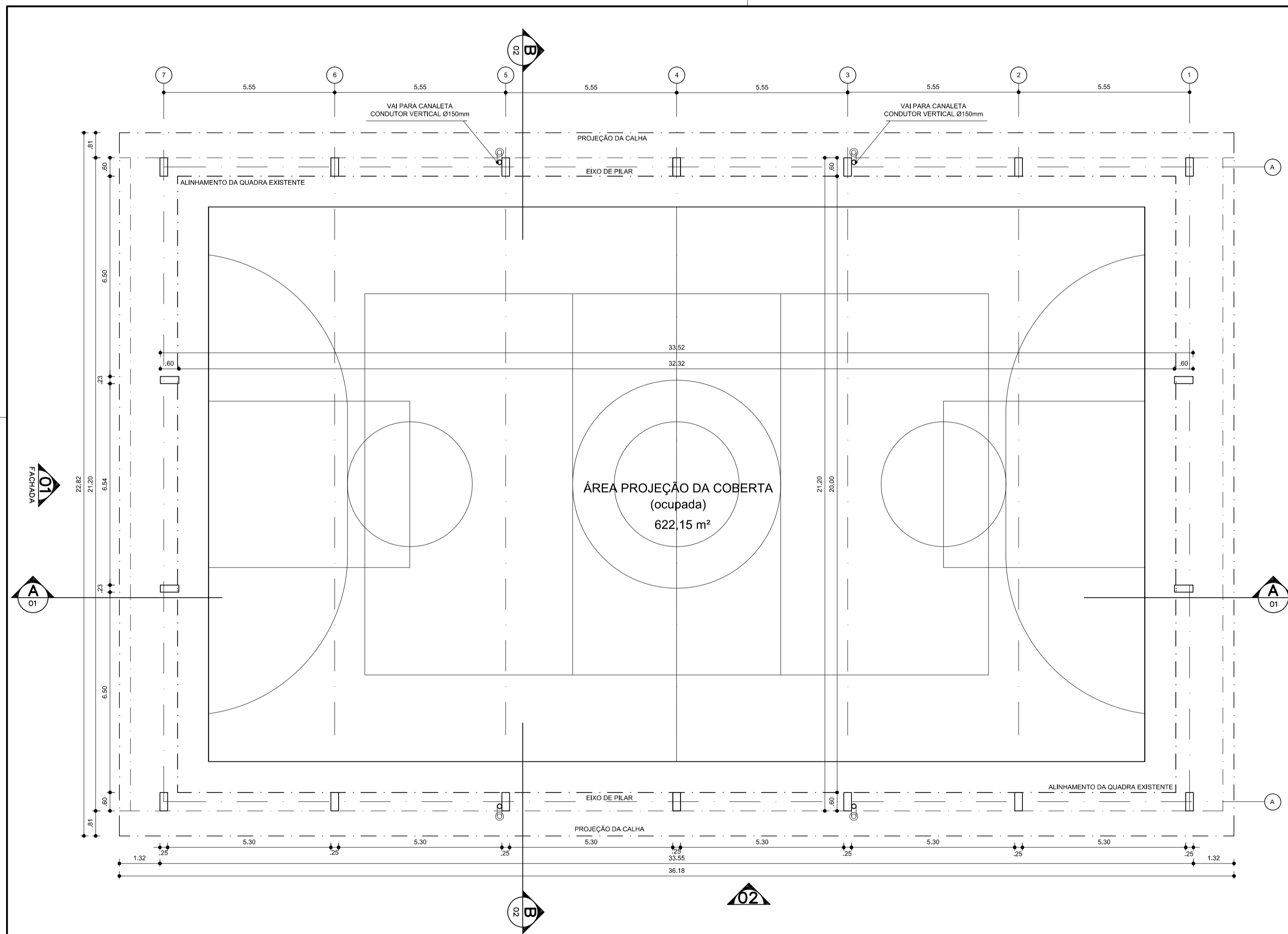
ARQ 01/07 PLANTA – BAIXA ESCALA 1/100
